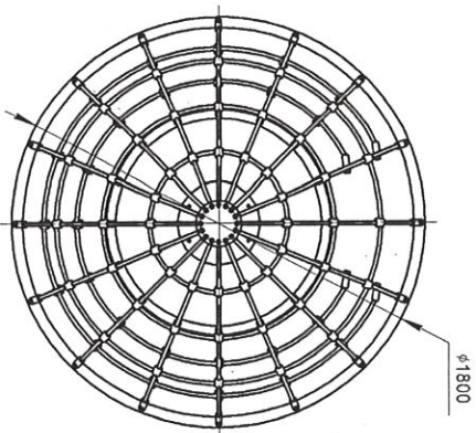
Рисунок 2 - Вид сверху
